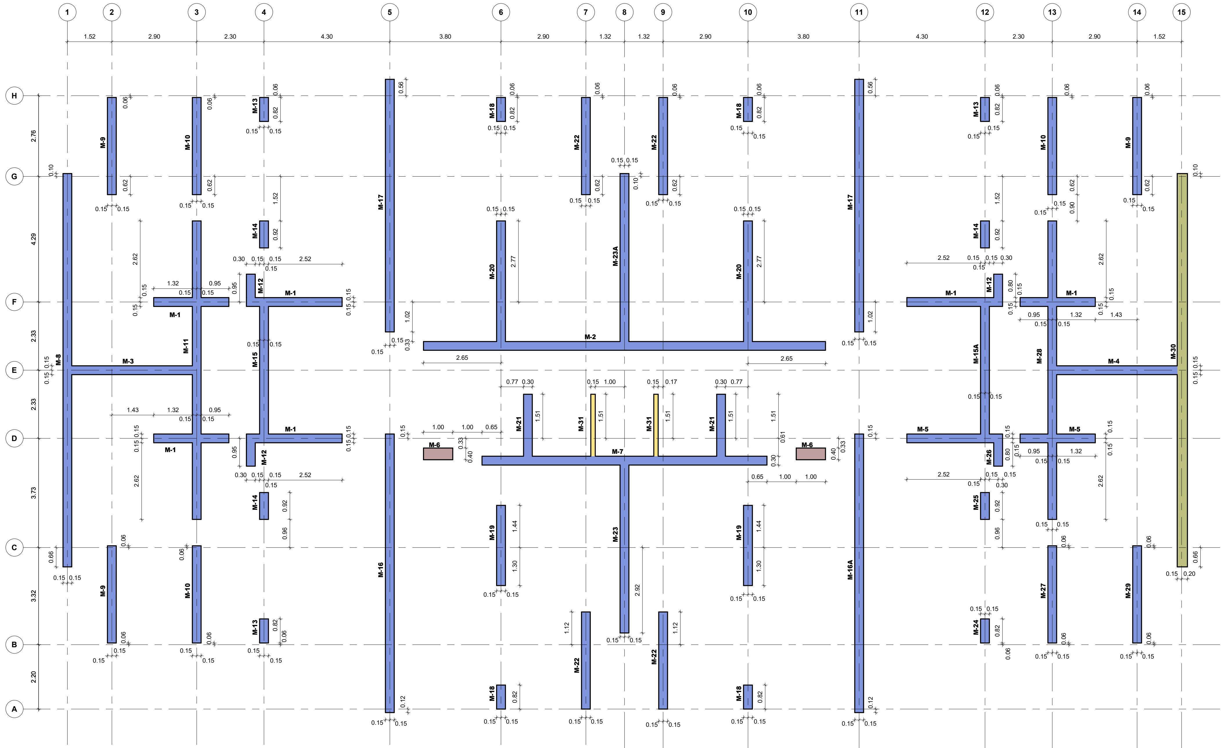
PLANTA LOCALIZACIÓN DE MUROS PISO 2 Escala 1 : 75
